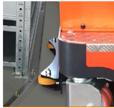
RL Führungsrollen.
